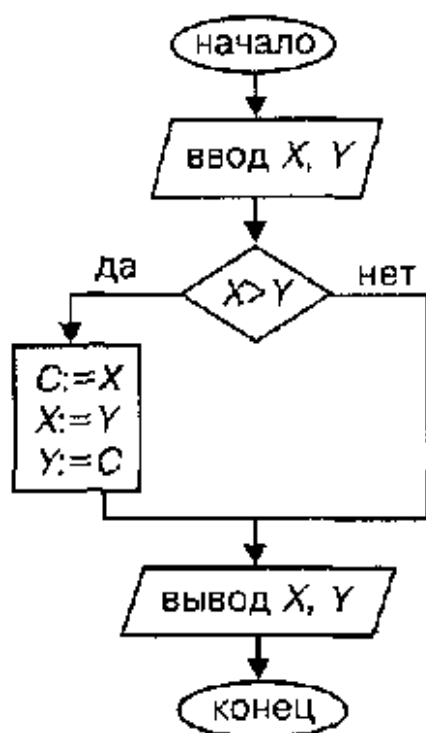
Рис. 6.4. Блок-схема алгоритма упорядочения двух величин
