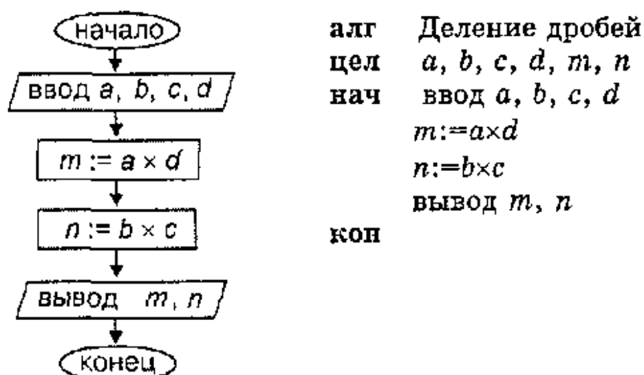
Рис. 6.1. Алгоритм деления дробей
