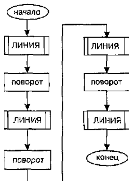
Рис. 5.8. Блок-схема алгоритма «Рамка»
