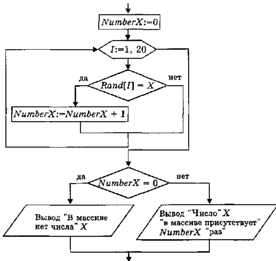
Рис. 6.11. Подсчет вхождений числа в массив
