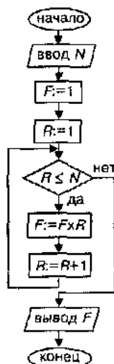
Рис. 6.7. Блок-схема алгоритма вычисления факториала
