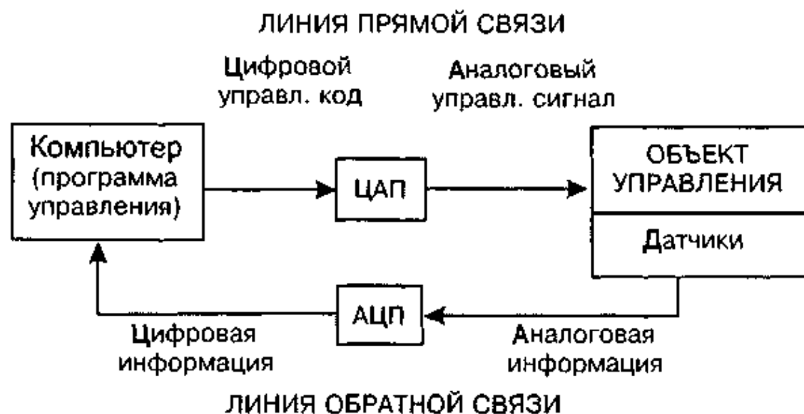
Рис. 5.16. Схема системы автоматического управления
